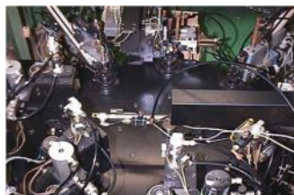
<メカスイッチ自動組立装置>
